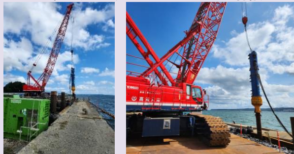
近畿地方 フライング油圧ハンマー打設
